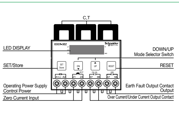
■ Hole Type
